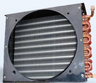
Condensor
